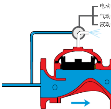
阀门开启（工作状态）
