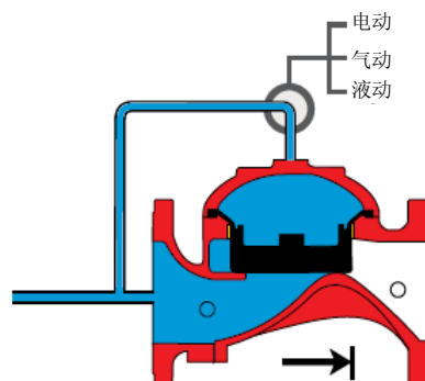
阀门关闭（设定位置）
