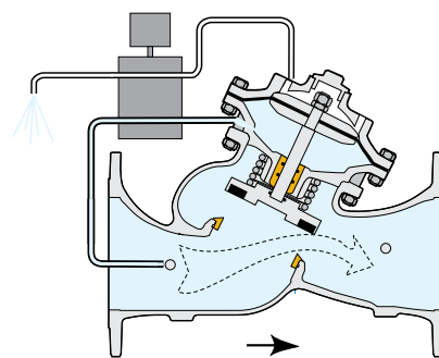
Позиция "Открыт гидравлическим усилием"
