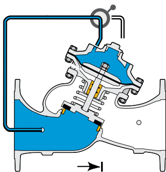
Позиция "Закрит"
