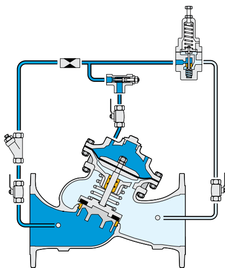
Позиция "Закрит"
