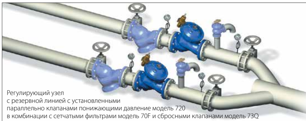
Регулирующий узел с клапаном понижающим и поддерживающим давление "до себя" модель 723 в комбинации с сетчатым фильтром модель 70F и сбросным клапаном модель 73Q
