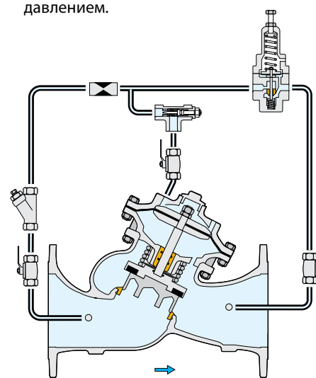
Позиция "Открыт"
