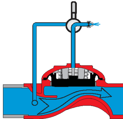
Válvula abierta
